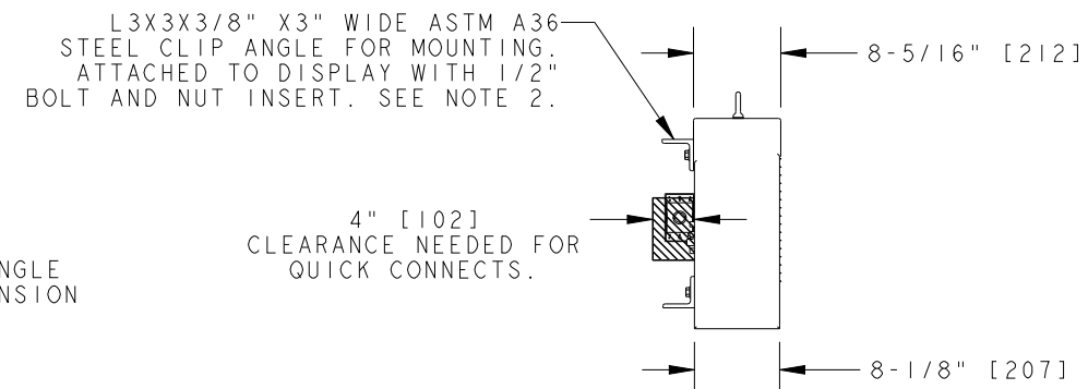
LEFT SIDE
