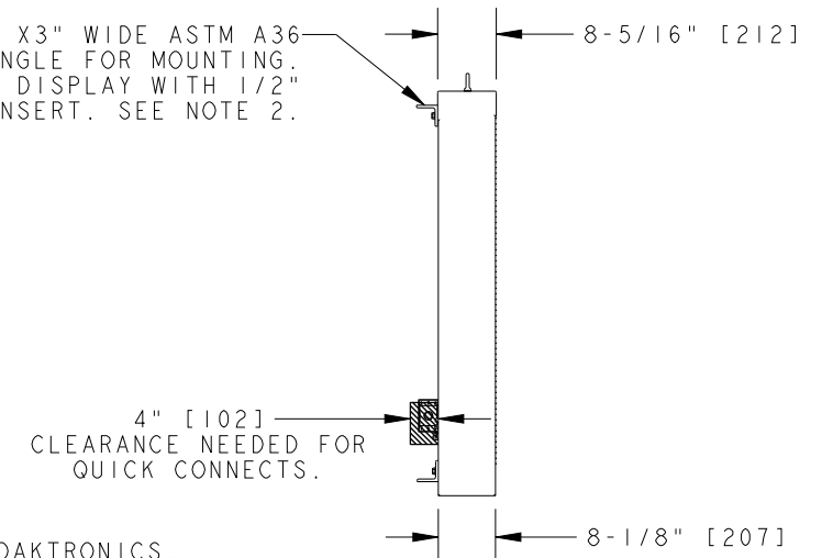
LEFT SIDE
