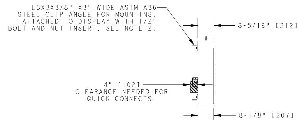
LEFT SIDE
